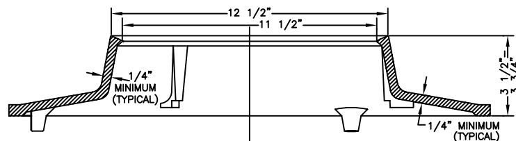
SECTION C-C LIGHT METER LID FRAME
